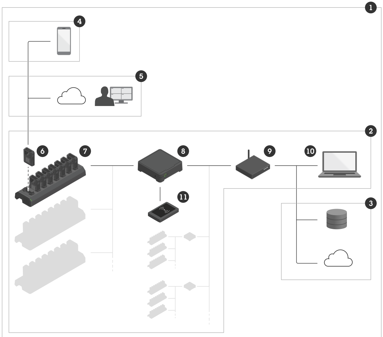
La soluzione indossabile Axis
