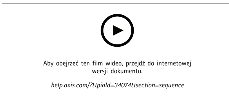
Dodawanie sekwencji
