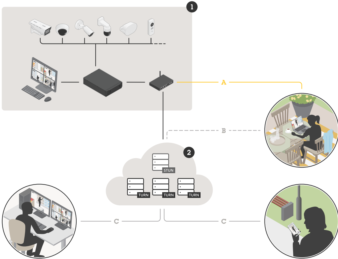
이미지: AXIS Camera Station Pro의 SRA v2 솔루션 개요
