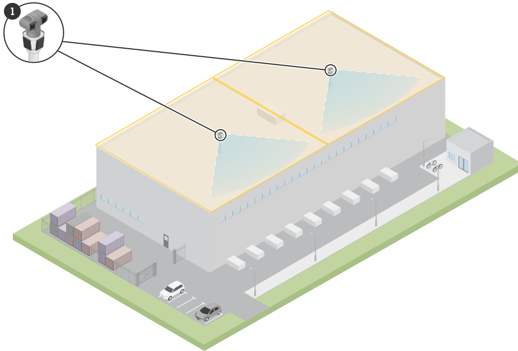
1 AXIS Q6225-LE PTZ Camera와 페어링된 AXIS D2124-VE Radar
