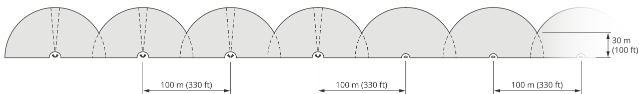
Quatre paires de radars AXIS D2210-VE et plusieurs AXIS D2110-VE Security Radars montés côte à côte.
