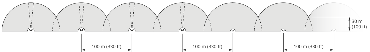
4쌍의 AXIS D2210-VE와 100m(330ft) 간격으로 설치된 여러 대의 AXIS D2110-VE Security Radar.
