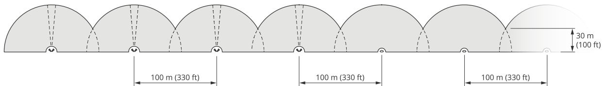
Quatro pares de AXIS D2210-VE e vários AXIS D2110-VE Security Radars montados com um espaçamento de 100 m (330 pés) entre eles.
