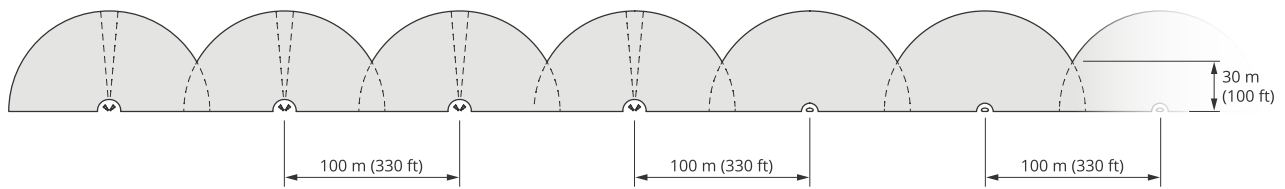
四对AXIS D2210-VE和多台AXIS D2110-VE Security Radar，安装间距100米（330英尺）。
