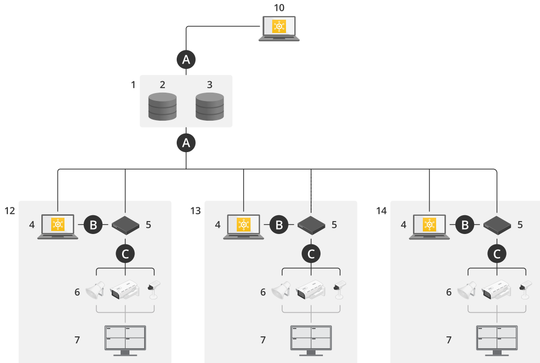
AXIS Device Manager Extender con acceso local y remoto usando una conexión VPN
