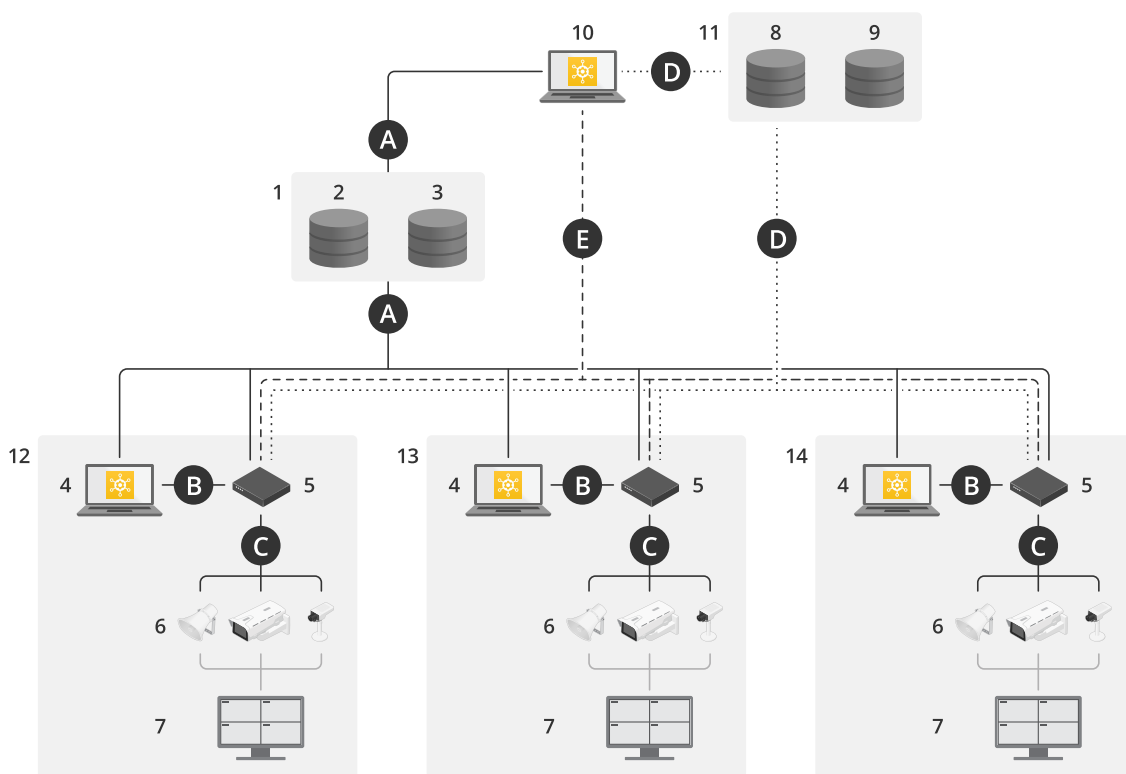
AXIS Device Manager Extend w konfiguracji wielostanowiskowej z wykorzystaniem lokalnego i zdalnego dostępu
