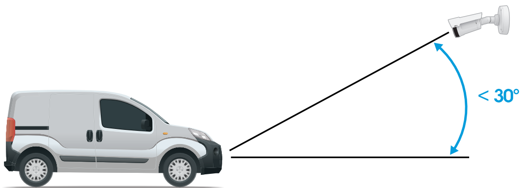
Montagewinkel von der Seite
