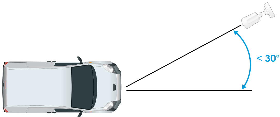
Angle de montage montré ci-dessus.
