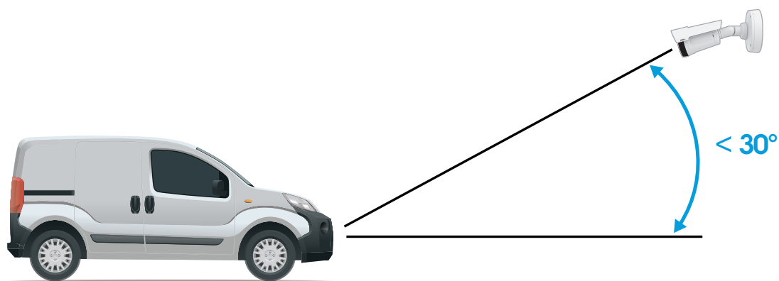
Ángulo de montaje desde el lateral.
