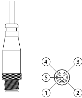
Connettore a 5 pin CC
