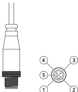
5ピンDCコネクタ
