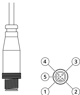
5 针 DC 连接器
