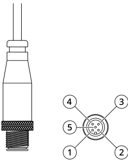
5-poliger DC-Anschluss
