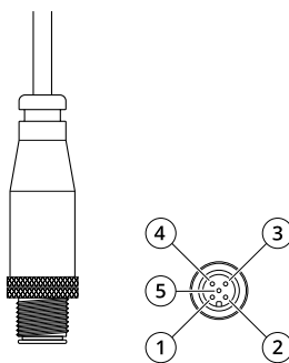
Conector de CC macho de 5 pines con código A
