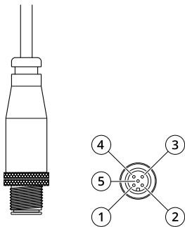
Connecteur CC à 5 broches
