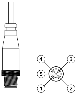
Connettore a 5 pin CC
