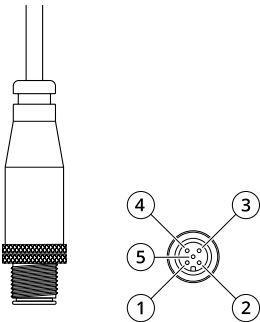
5ピンDCコネクター
