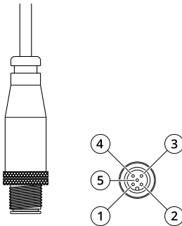
5핀 메일 A-코드 DC 커넥터
