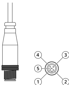
5핀 메일 A-코드 DC 커넥터
