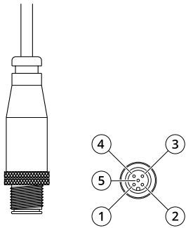
5 針 DC 接頭
