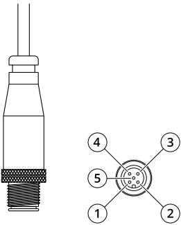
5 針 DC 接頭
