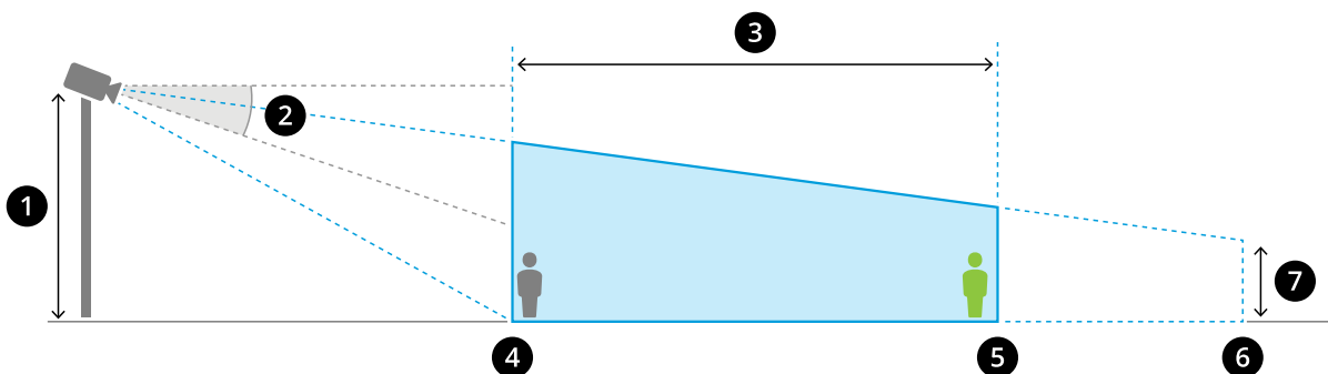
Eine ordnungsgemäß installierte Kamera.
