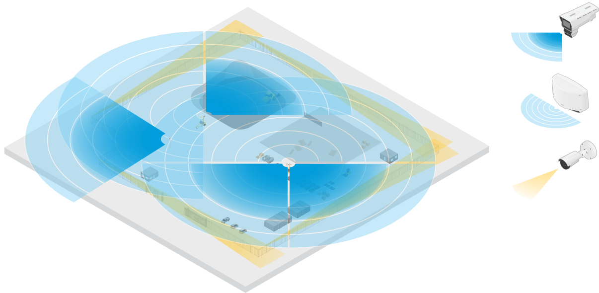
Exemple de chantier de construction où deux radars autonomes couvrent les zones ouvertes du site tandis que quatre caméras de fusion radar-vidéo couvrent les zones ouvertes les plus complexes. En outre, quatre caméras thermiques couvrent les couloirs étroits le long de la clôture.
