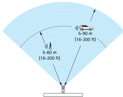
Erfassungsbereiche für Personen und Fahrzeuge mit dem Profil „Bereichsüberwachung“.
