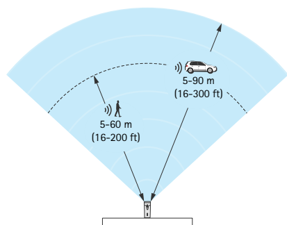
Rangos de detección de personas y vehículos con el perfil de supervisión de área.
