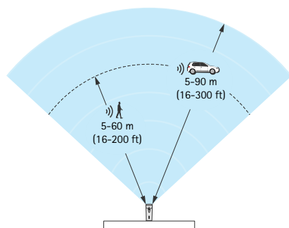
Plages de détection pour les êtres humains et les véhicules avec le profil de surveillance de zone.
