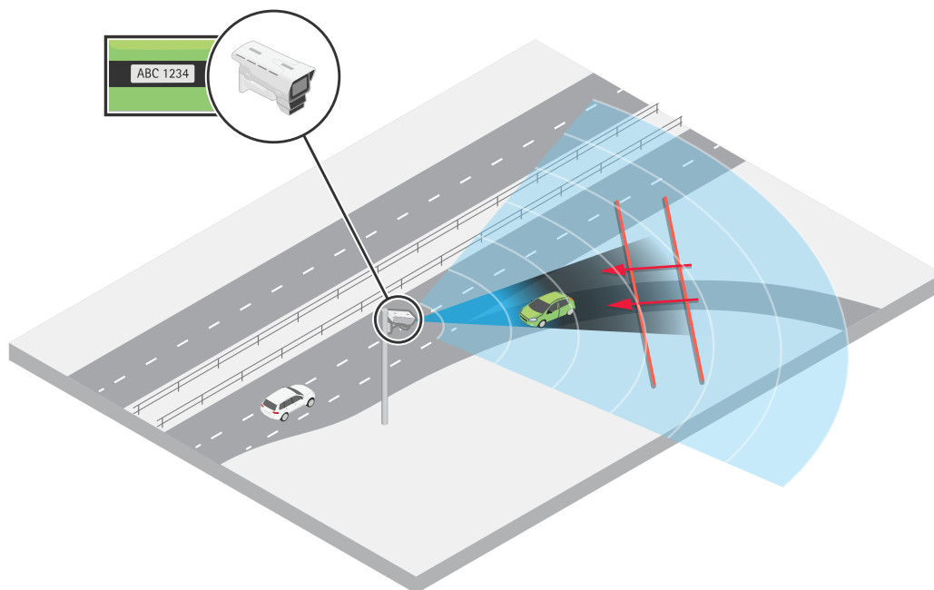
Detekcja jazdy w niewłaściwym kierunku w przypadku pojazdów zbliżających się
