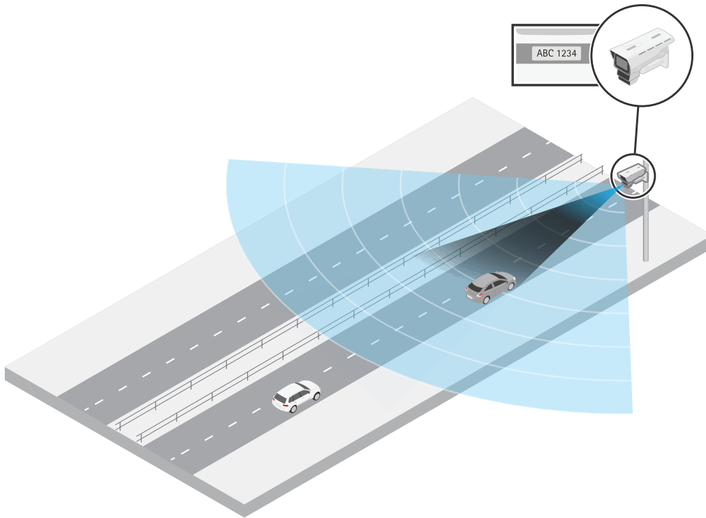
AXIS Q1686-DLE 安装在高速公路一侧的一根立杆上，可测量正在接近的车辆的速度并抓取牌照。
