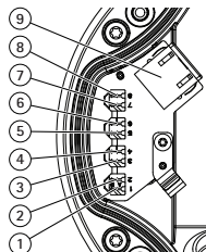
1-8 IDCコネクタ 9 パッチケーブルコネクタ
