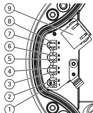
1-8 IDCコネクター 9 パッチケーブルコネクター
