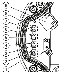
1-8 Conectores IDC 9 Conector do cabo de patch
