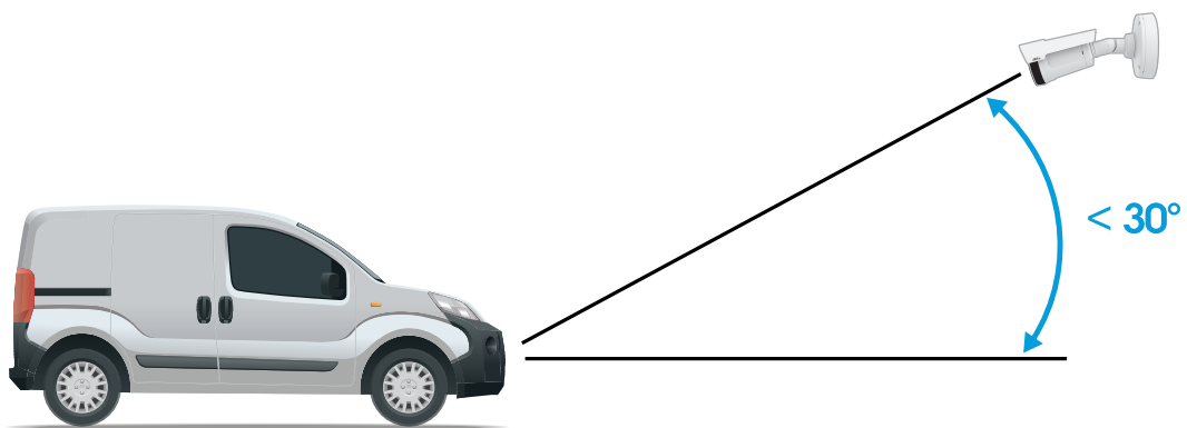
横からの取り付け角度。
