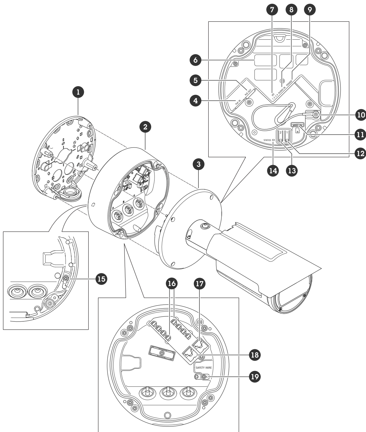
1 安裝支架
