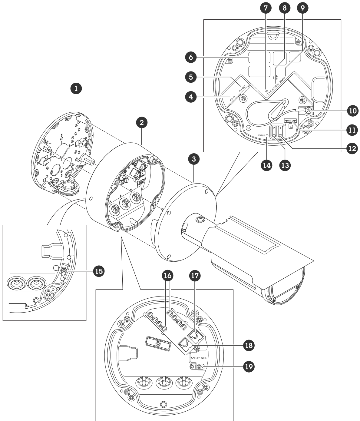
1 Uchwyt montażowy
