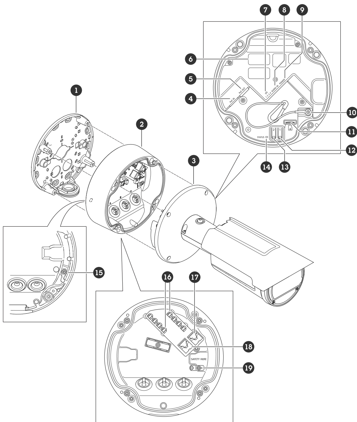
1 安装支架
