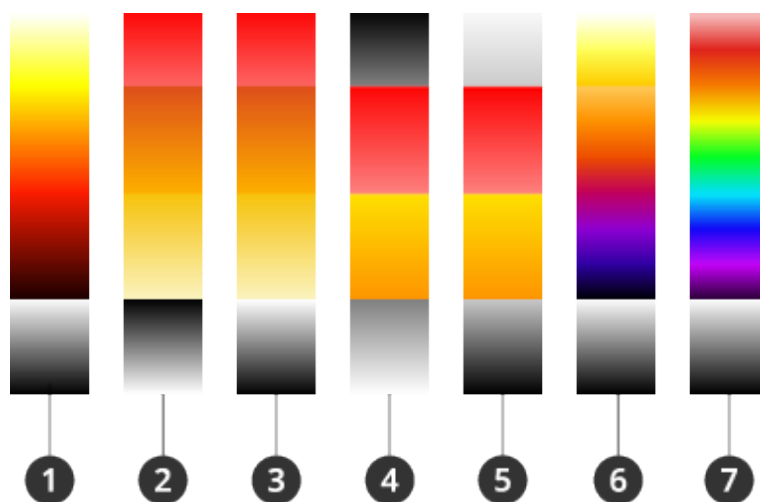
Palettes isothermes
