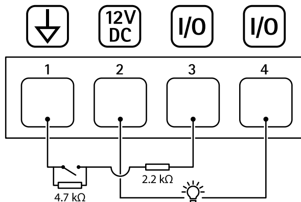
1 Erdung Gleichstrom
