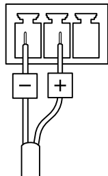
DC 电源输入
