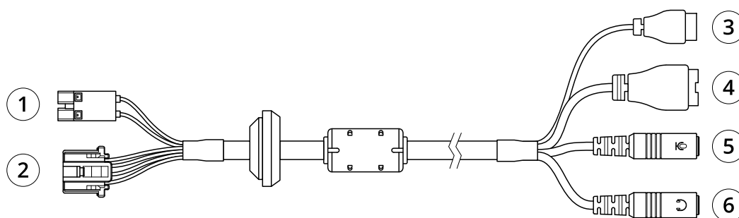
Opis kabla wielofunkcyjnego
