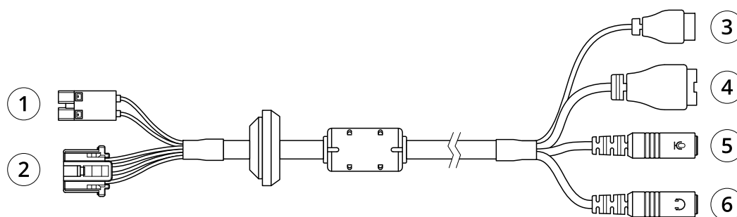
マルチケーブルの概要
