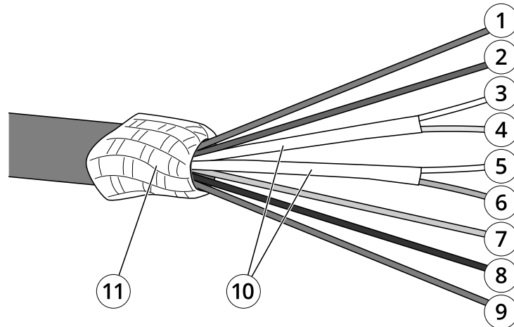
Übersicht Mehrfachkabel
