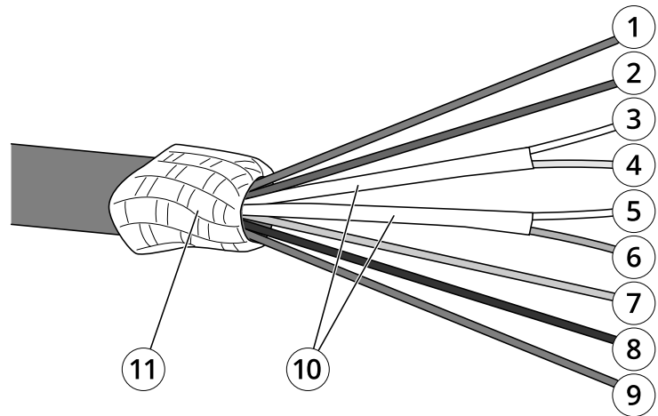
多芯电缆概览
