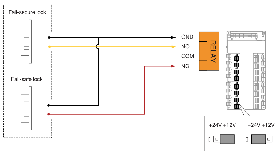
Relé de puerta
