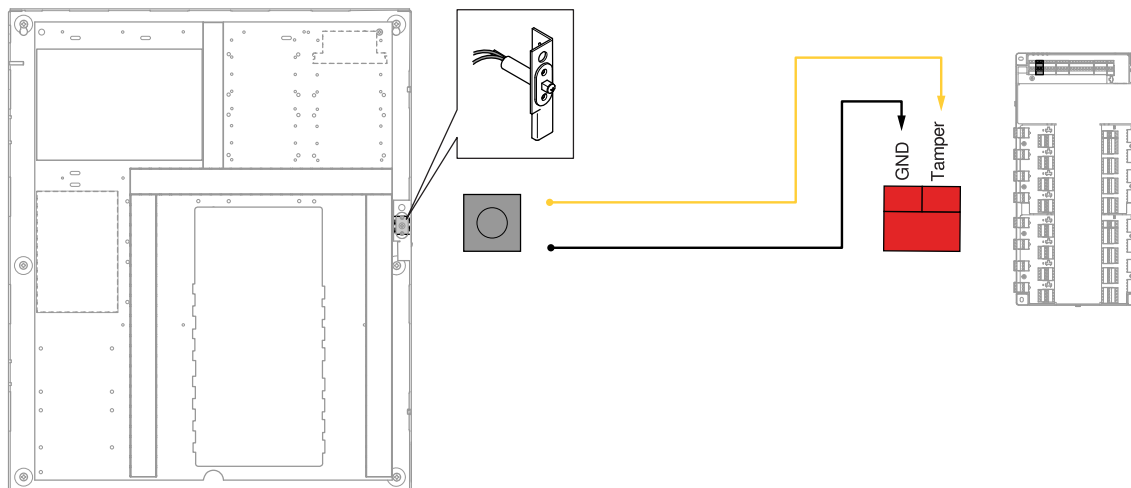
Interruptor de manipulación al controlador de puerta
