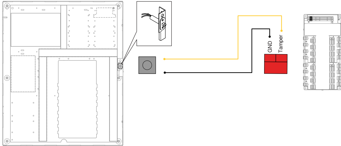
Interrupor de manipulación al controlador de puerta
