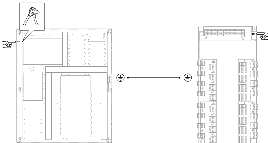
Controlador de puerta a tierra de la carcasa
