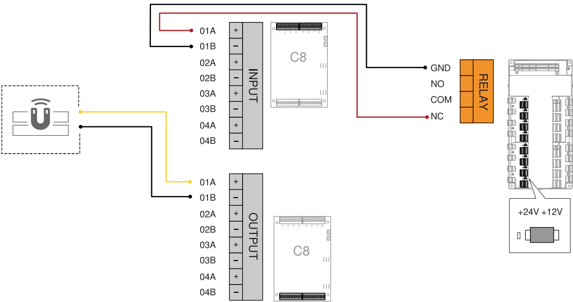
Relé de puerta a C8, opción 2
