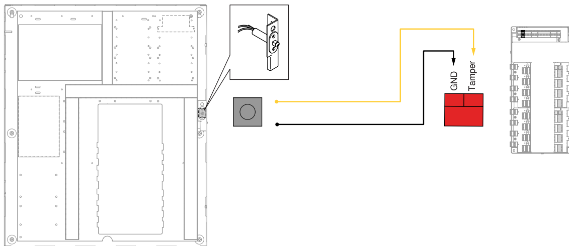
Interrupteur anti-sabotage vers le contrôleur de porte
