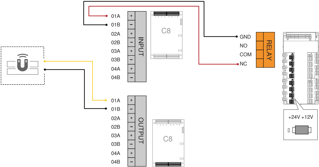
Relais de porte vers C8, option 2
